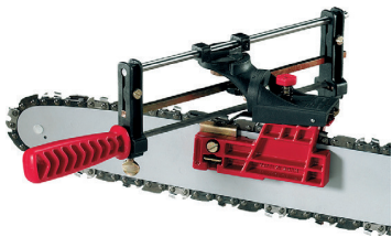
Afiladora de cadena TECOMEC 0020350
